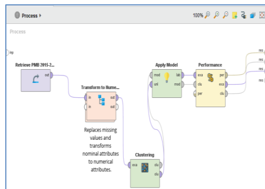
Gambar 6. Desain Clustering Menggunakan Algoritma K-Medoids
