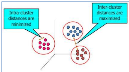
Gambar 2. Konsep Clustering (Han, 2006)
