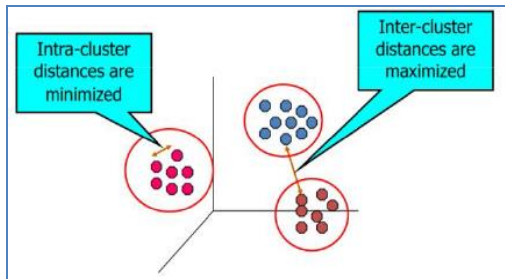
Gambar 4. Konsep Clustering [9]
